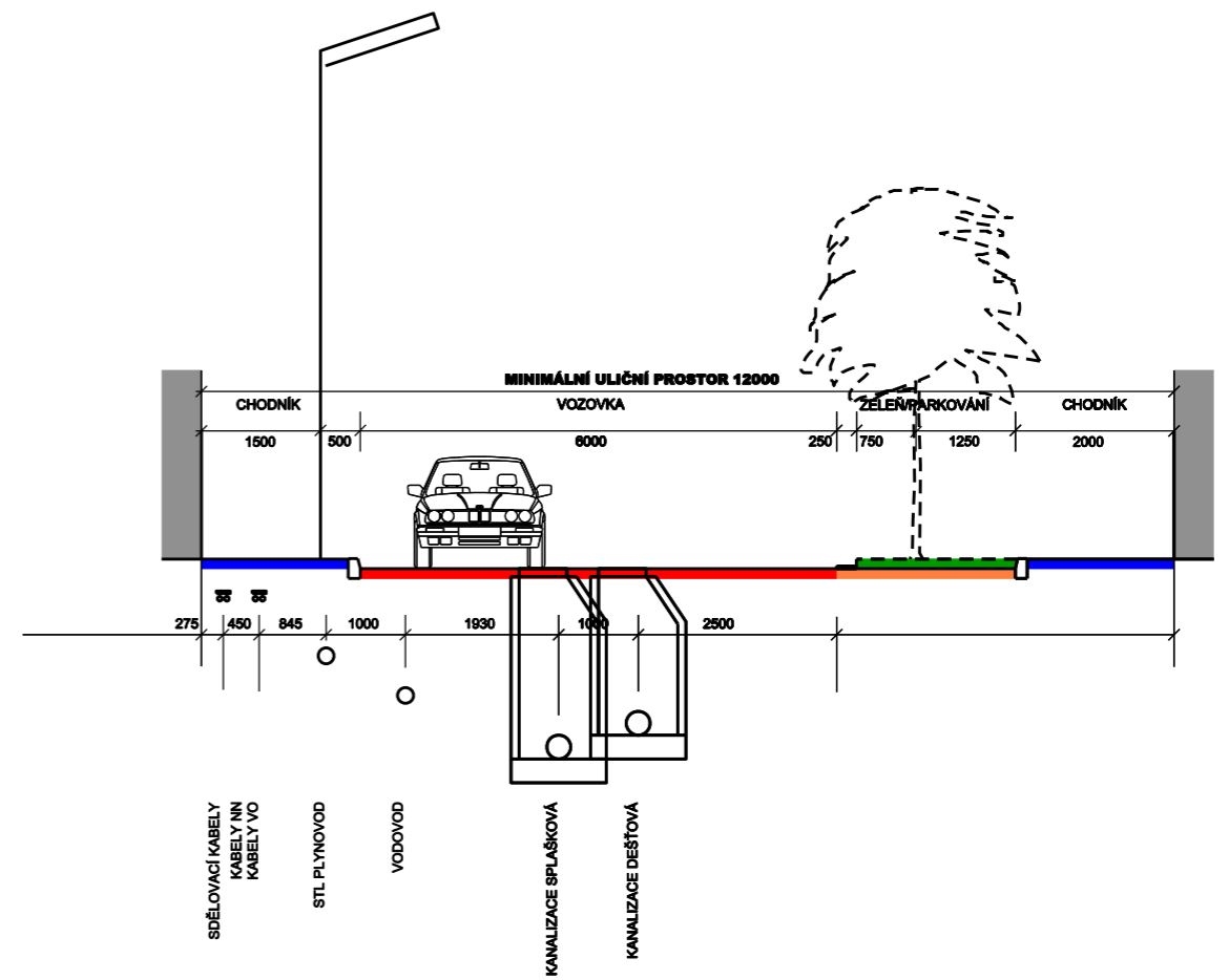
CHARAKTERISTICKÝ PŘÍČNÝ ŘEZ KOMUNIKACÍ 1:100 ULIČNÍ PROFIL "C" - SLADOVNICKÁ PODEL RD
