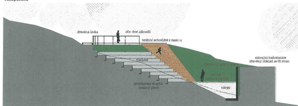
řezopohled
