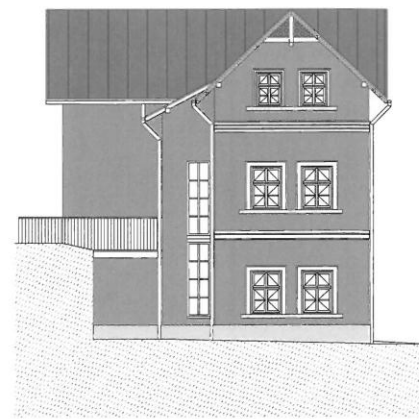
pohled jihovýchodní
