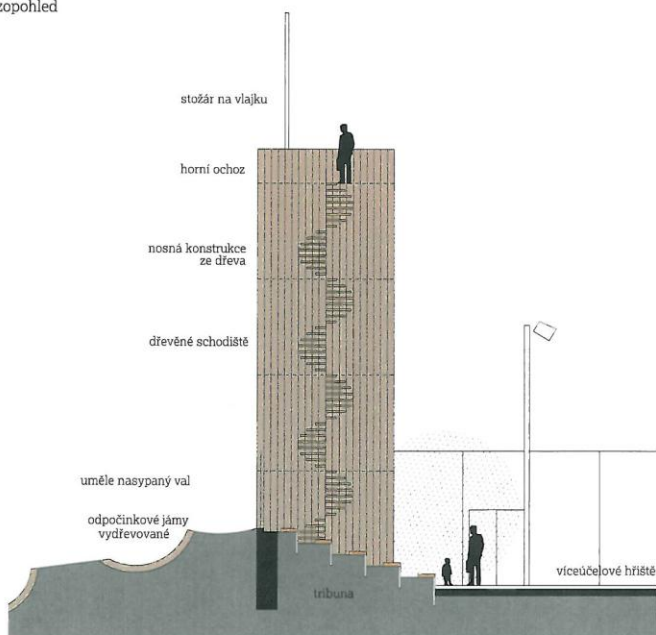
řezopohled
