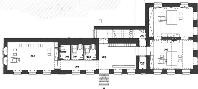
půdorys 1.n.p.
