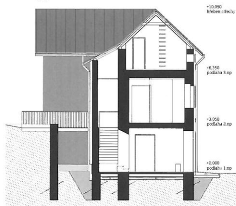
řez
