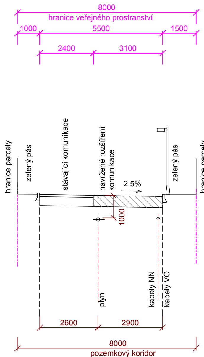
Schematický řez komunikací hlavní - ul. Dubová chodník 1.5m + komunikace - š.5,5m + zelený pás š.1,0m
