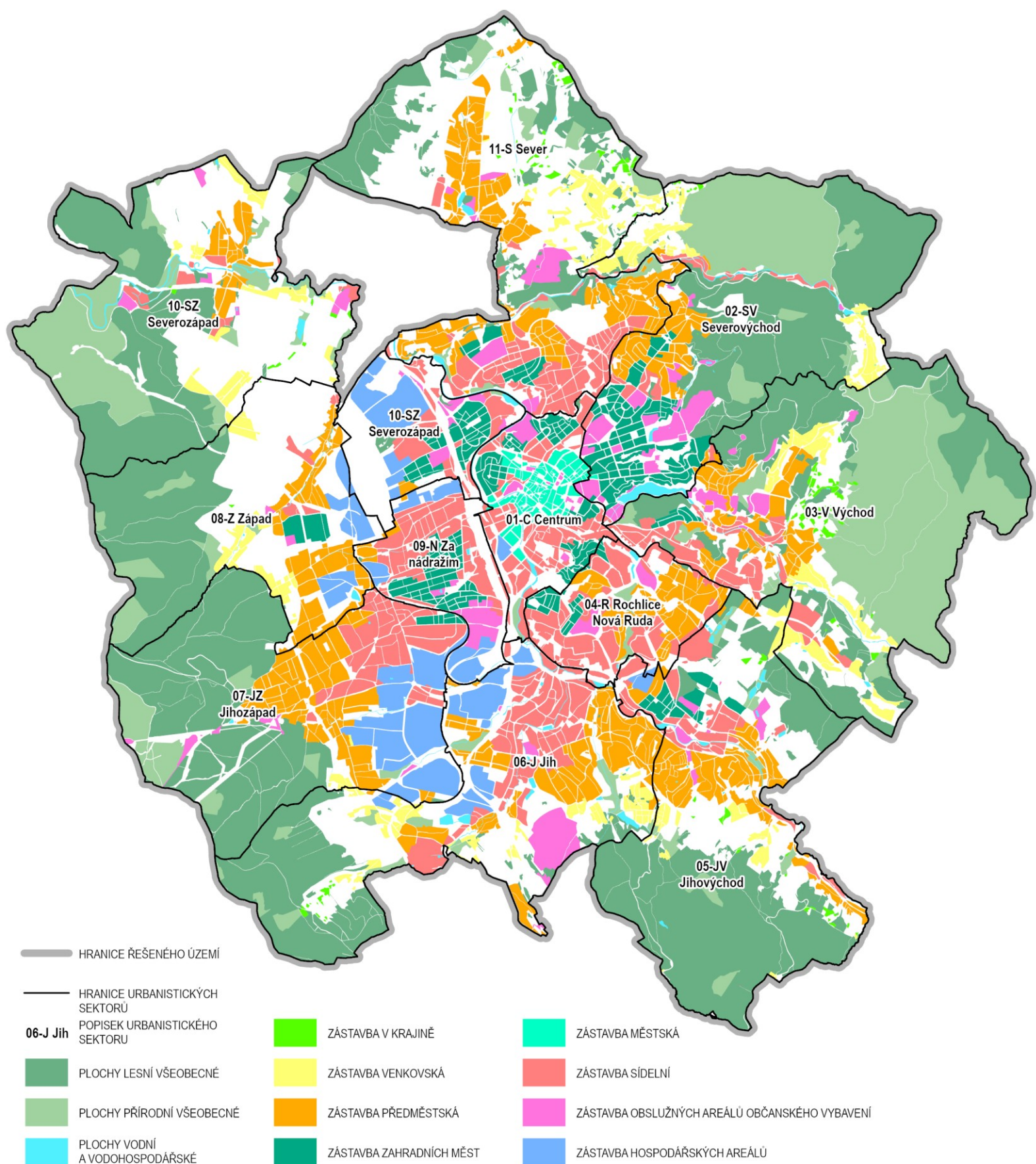
SCHÉMA F.4.4 CHARAKTER ZÁSTAVBY
