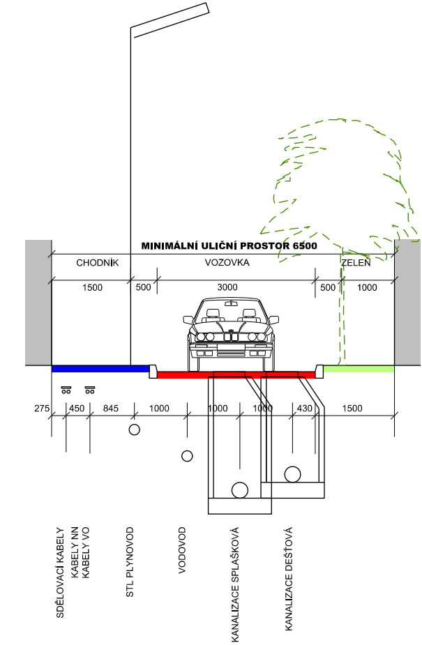
CHARAKTERISTICKÝ PŘÍČNÝ ŘEZ KOMUNIKACÍ 1:100 ULIČNÍ PROFIL "C" PŘÍSTUPOVÁ JEDNOSMĚRNÁ
