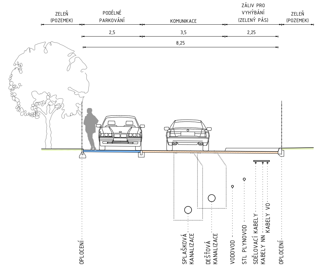
SCHEMATICKÝ PŘÍČNÝ ŘEZ MÍSTNÍ KOMUNIKACÍ - VEDLEJŠÍ MO1 8/3,5/20
