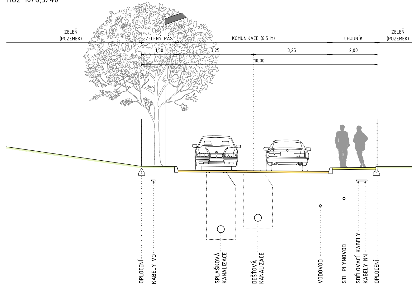
SCHEMATICKÝ PŘÍČNÝ ŘEZ MÍSTNÍ KOMUNIKACÍ - HLAVNÍ MO2 10/6,5/40
