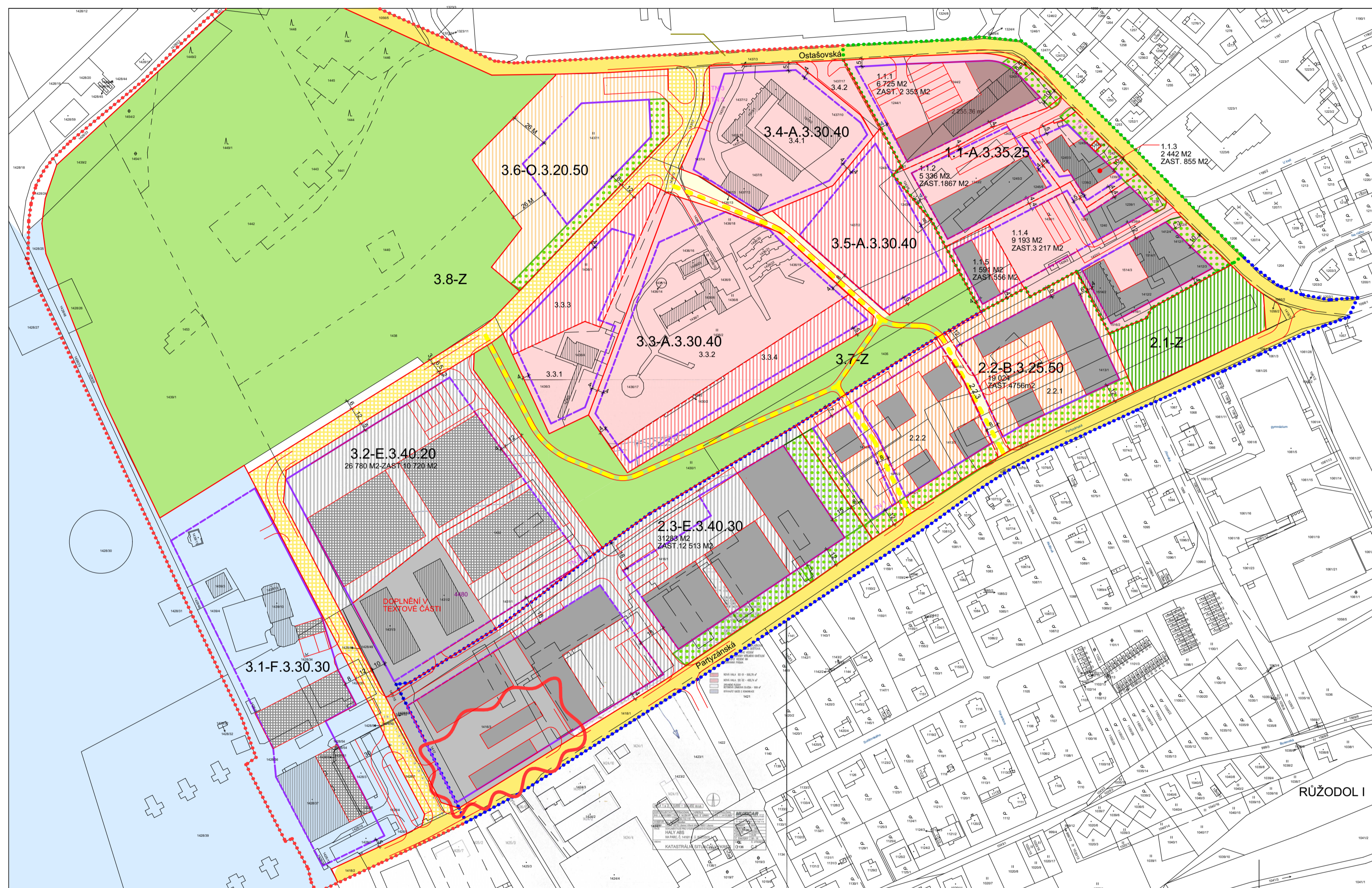
HLAVNÍ VÝKRES - SITUACE 1:2000
