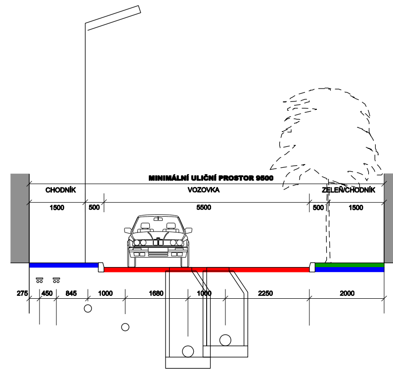
CHARAKTERISTICKÝ PŘÍČNÝ ŘEZ KOMUNIKACÍ 1:100 ULIČNÍ PROFIL "C" PŘÍSTUPOVÁ OBOUSMĚRNÁ
