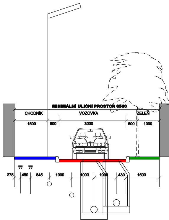
CHARAKTERISTICKÝ PŘÍČNÝ ŘEZ KOMUNIKACÍ 1:100 ULIČNÍ PROFIL "C" PŘÍSTUPOVÁ JEDNOSMĚRNÁ
