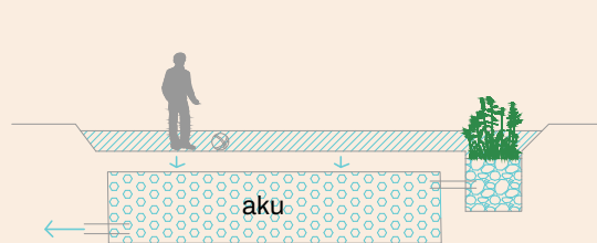
6. pobytový retenční průleh s půdním filtrem a akumulační nádrží
