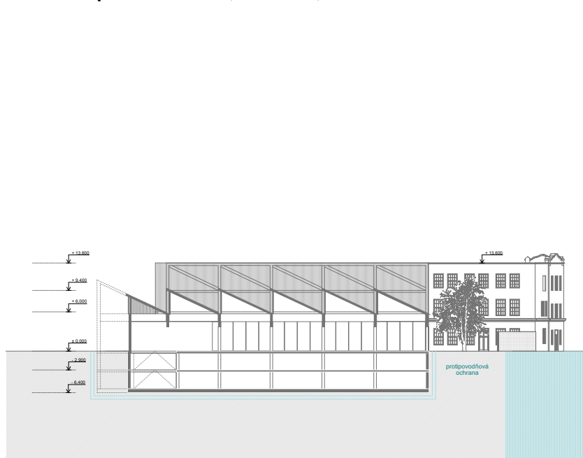
Řez AA'
